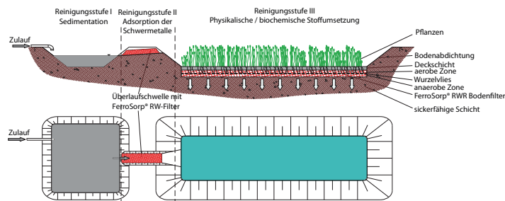
Einsatz von FerroSorp® RW bei der offenen Regenwasserversickerung mit vorgeschalteter Sedimentation
