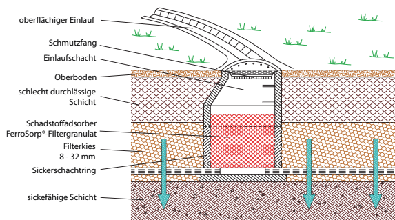
Einsatz von FerroSorp® RW bei der Schachtvorsickerung
